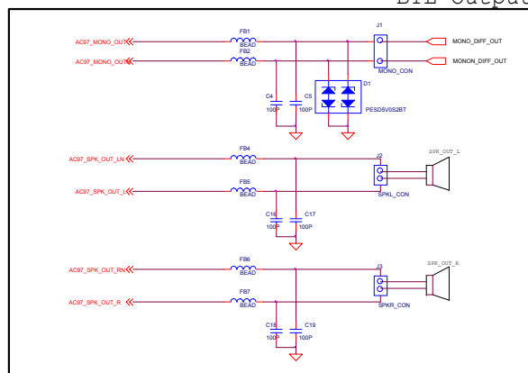
BTL Output
