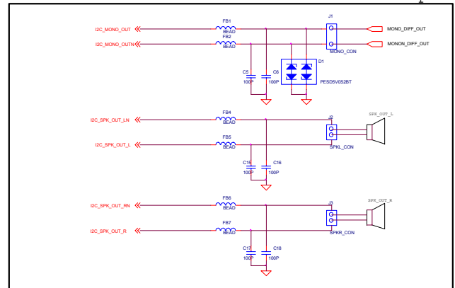
BTL Output
