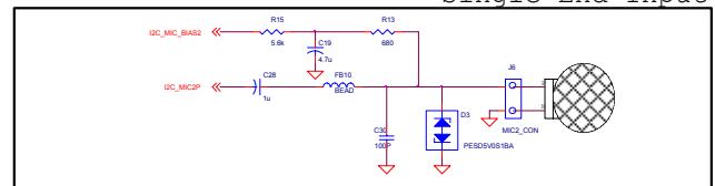
Analog Stereo Input
